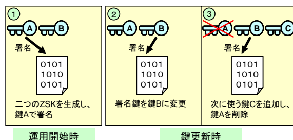
図2:ZSK の更新手順例(事前公開法)
